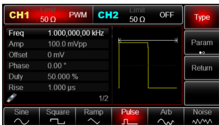
Рис. 88 Настройка параметров несущего сигнала
