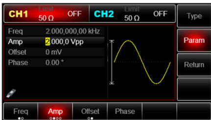
Рис. 65 Установка амплитуды несущего сигнала
