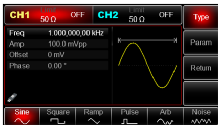
Рис. 68 Выбор формы несущего сигнала
