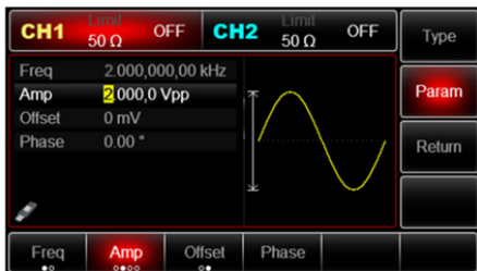
Рис. 60 Установка амплитуды несущего сигнала
