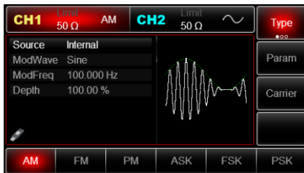
Рис. 20 Амплитудно-модулированный сигнал
