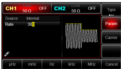
Рис. 46 Установка частоты следования прямоугольных импульсов в режиме ASK
