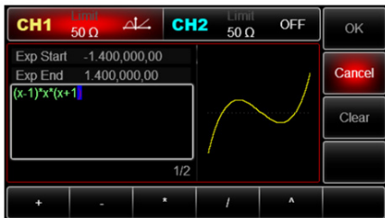
Рис. 18 Задание функции сигнала пользователем
