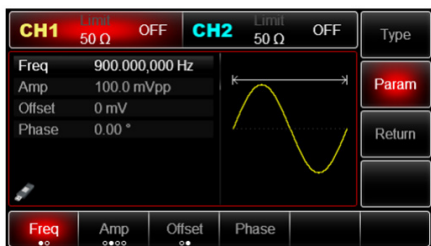
Рис. 40 Установка параметров несущего сигнала
