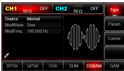
Рис. 77 Параметры модулирующего сигнала в режиме DSBAM
