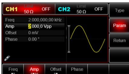
Рис. 69 Установка амплитуды несущего сигнала
