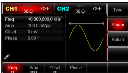
Рис. 33 Выбор параметров несущего сигнала
