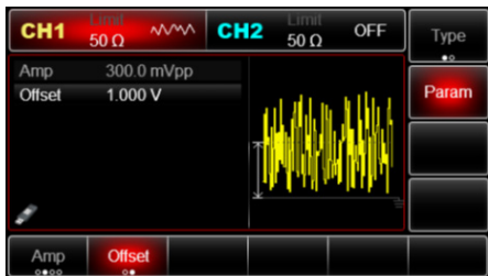
Рис. 15 Установка параметров шумового сигнала
