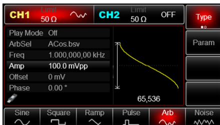
Рис. 119 Выберите функцию произвольной формы
