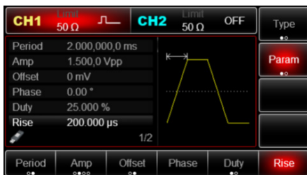
Рис. 12 Установка параметров импульсного сигнала
