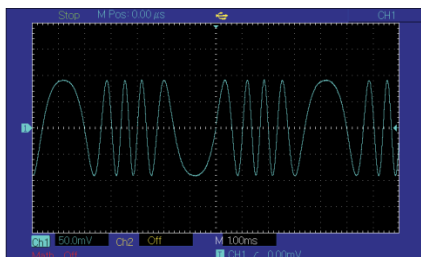
Рис. 42 Осциллограмма сформированного фазо-модулированного сигнала
