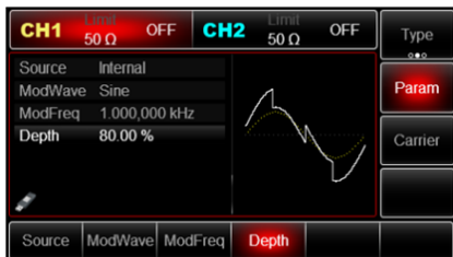
Рис. 74 Установка глубины модуляции в режиме модуляции SUM
