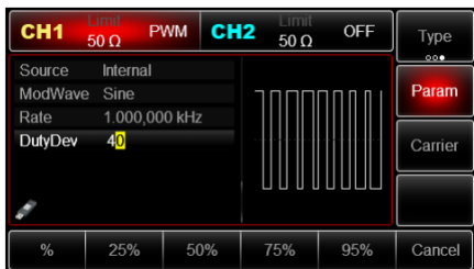
Рис. 91 Установка девиации коэффициента заполнения импульсов
