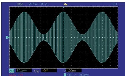
Рис. 28 Осциллограмма сформированного амплитудно-модулированного сигнала
