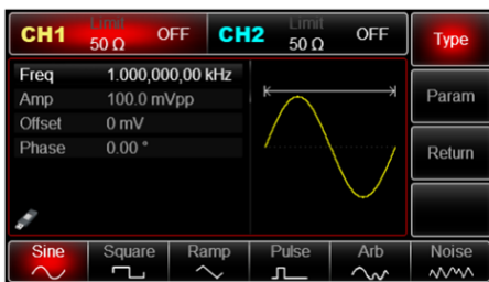
Рис. 59 Выбор формы несущего сигнала
