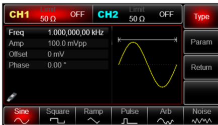
Рис. 49 Выбор формы несущего сигнала
