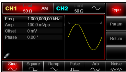
Рис. 76 Настройка параметров несущего сигнала
