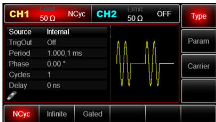
Рис. 108 Режим N-цикла
