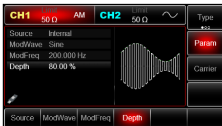
Рис. 27 Амплитудно-модулированный сигнал с глубиной модуляции 80 %
