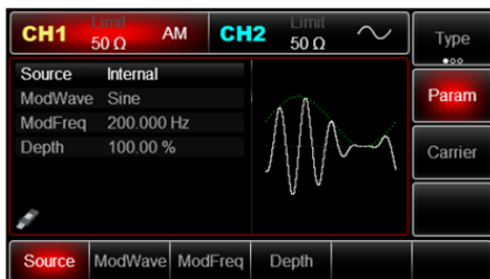
Рис. 23 Установка параметров модулирующего сигнала в режиме AM
