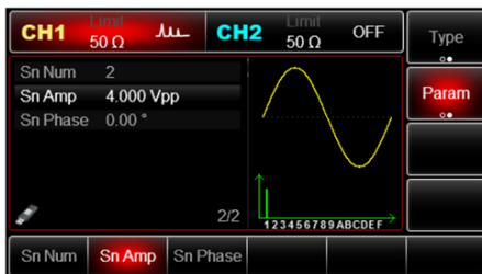
Рис. 16 Настройка кратных гармоник сигнала
