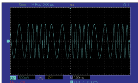
Рис. 52 Осциллограмма сформированного частотно-манипулированного сигнала
