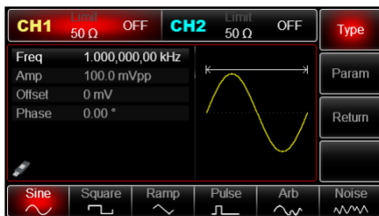
Рис. 32 Выбор формы несущего сигнала
