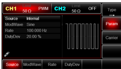
Рис. 89 Установка параметров модулирующего сигнала в режиме PWM
