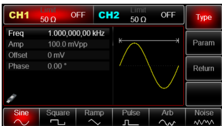
Рис. 39 Выбор формы несущего сигнала
