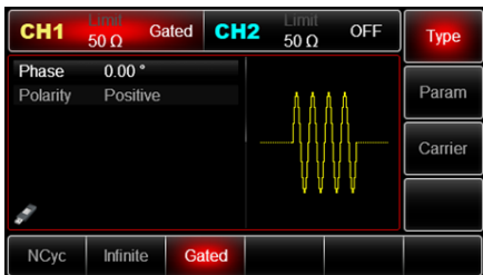
Рис. 109 Режим стробирования
