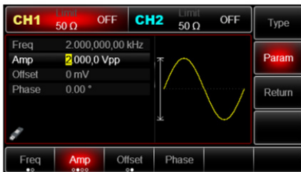
Рис. 79 Установка амплитуды несущего сигнала в режиме DSBAM
