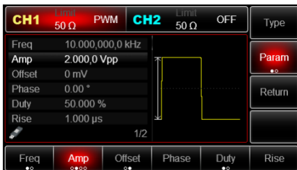
Рис. 90 Установка параметров несущего сигнала в режиме PWM
