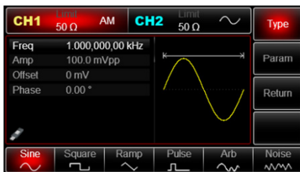
Рис. 83 Настройка параметров несущего сигнала
