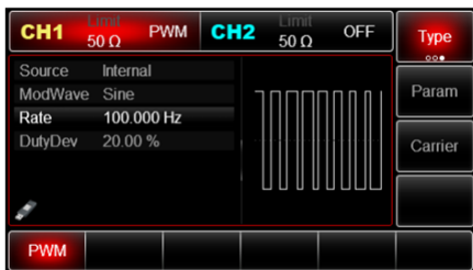
Рис. 87 Выбор широтно-импульсной модуляции (PWM) в списке доступных видов модуляции
