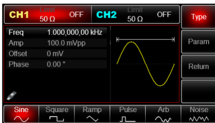
Рис. 44 Выбор формы несущего сигнала
