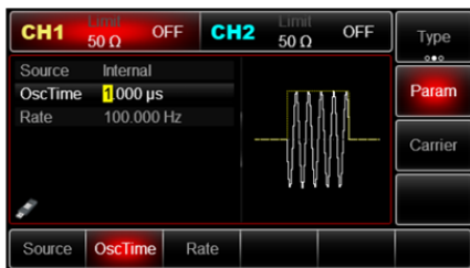
Рис. 70 Установка периода колебания, генерируемого внутренним опорным генератором, в режиме OSK
