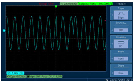
Рис. 66 Осциллограмма сформированного сигнала QPSK
