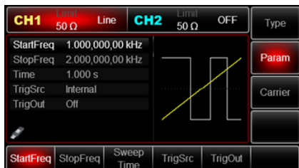
Рис. 103 Установка начальной частоты запуска
