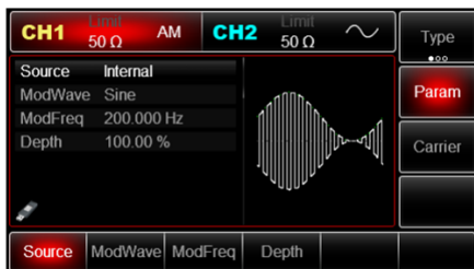
Рис. 26 Амплитудно-модулированный сигнал с глубиной модуляции 100 %
