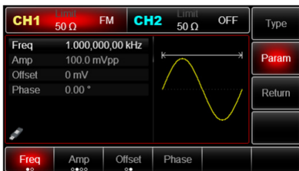
Рис. 36 Настройка параметров несущего сигнала
