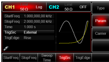
Рис. 98 Выбор внешнего источника запуска
