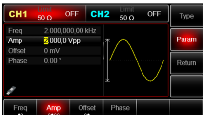
Рис. 55 Установка амплитуды несущего сигнала
