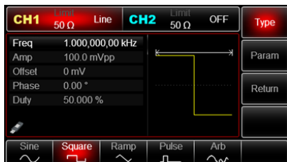
Рис. 100 Выберите форму сигнала частотной развёртки
