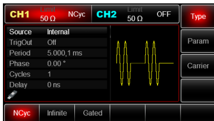
Рис. 115 Настройка параметров последовательности импульсов
