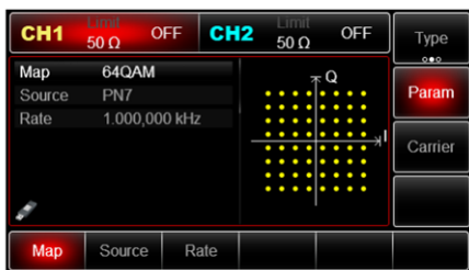
Рис. 85 Установка порядка квадратурной амплитудной модуляции
