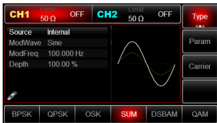
Рис. 72 Параметры суммирующей модуляции SUM
