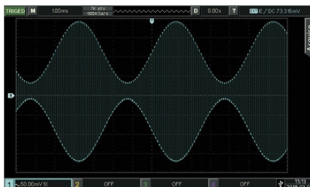
Рис. 11 Амплитудно-модулированный сигнал
