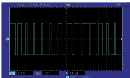
Рис. 92 Осциллограмма сформированного сигнала с широтно-импульсной модуляцией
