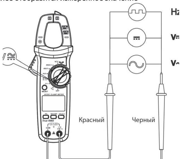
Рис. 3 Измерение напряжения переменного/постоянного тока и частоты
