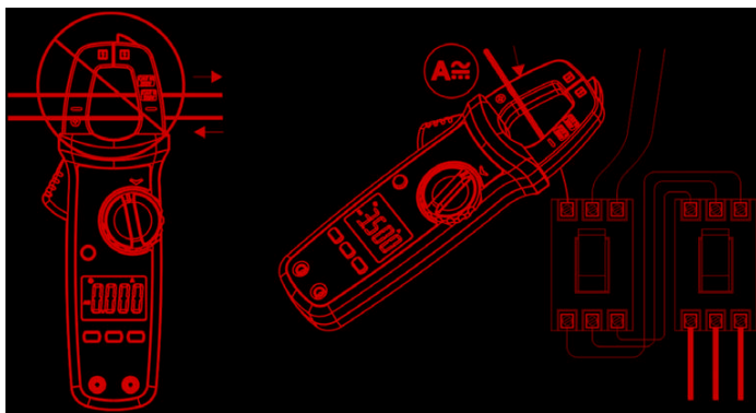
Рис. 2 Измерение силы переменного/постоянного тока
