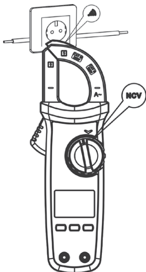
Рис. 5 Бесконтактное обнаружение переменного напряжения
