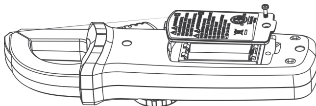
Рис. 7 Замена батареек
